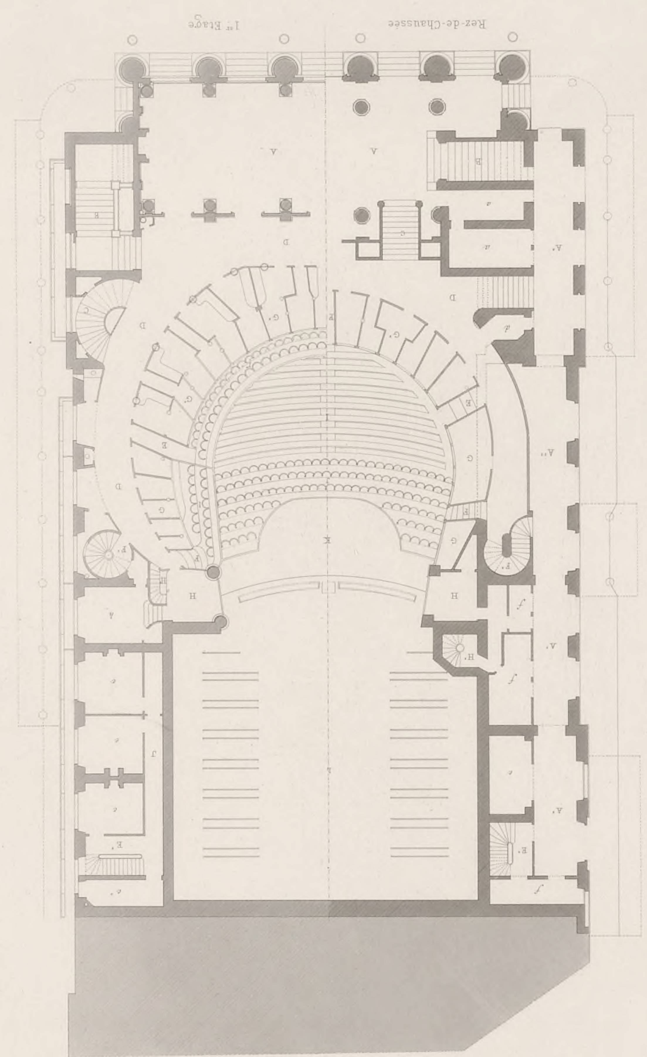
PLAN DU NOUVEAU THEATRE ROYAL DE L'OPERA COMIQUE. SALLE FAVART A PARIS
